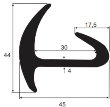
113279 SBR 80 Sh A Vedação porta container
