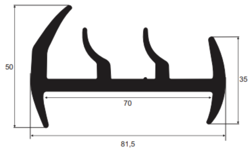
113305 EPDM 75 Sh A Vedação furgões frigoríficos Niju
