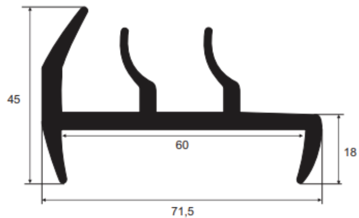
113538 EPDM 75 Sh A Vedação porta frigorífico
