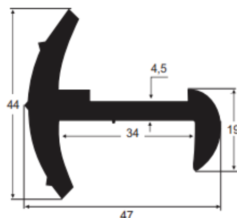
113223 SBR 85 Sh A Vedação porta furgões
