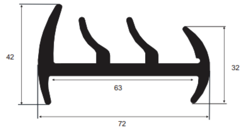
113693 EPDM 70 Sh A Vedação porta frigorífico
