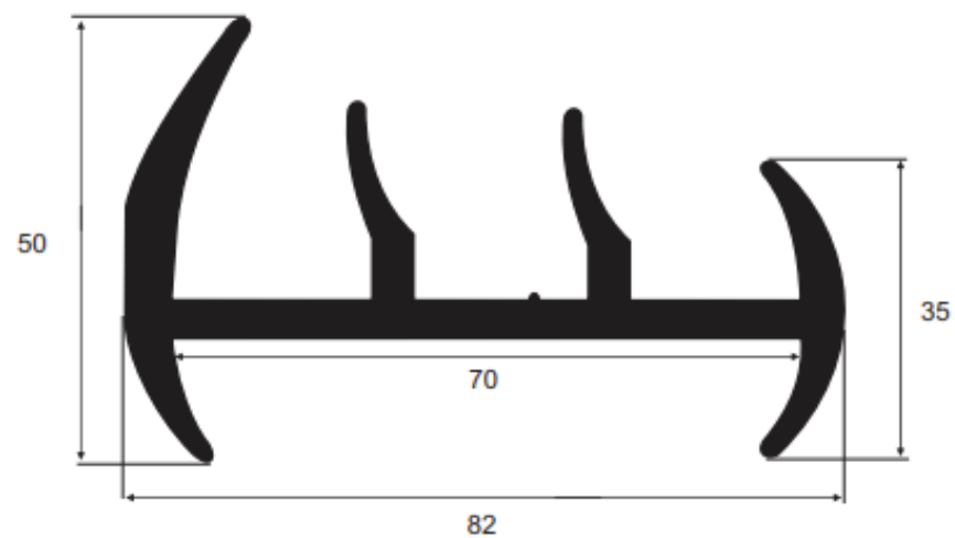
113379 EPDM 70 Sh A Vedação furgões frigoríficos Randon
