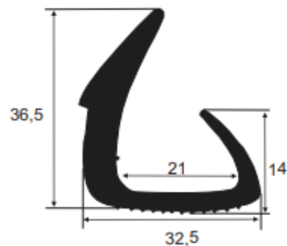
113277 SBR 80 Sh A Vedação porta container
