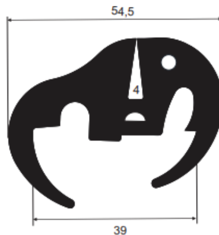
118051 SBR 60 Sh A Vedação cabine máq. agrícola
