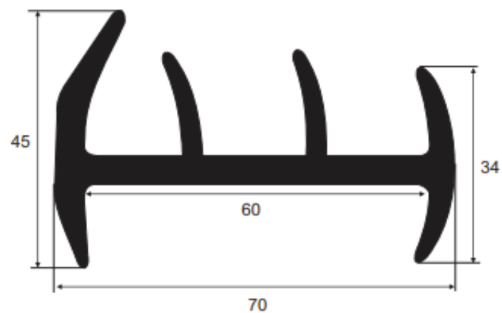
113536 EPDM 75 Sh A Vedação porta frigorífico
