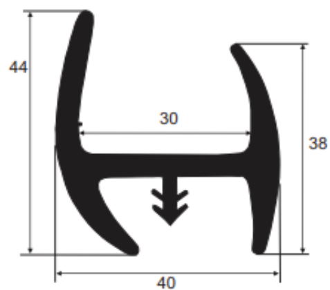
113278 SBR 80 Sh A Vedação porta container
