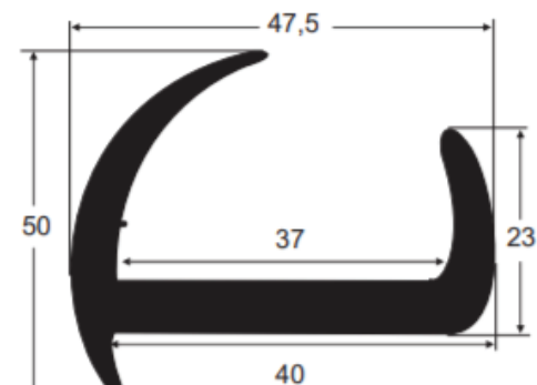
113205 SBR 80 Sh A 113451 EPDM 80 Sh A Vedação porta container
