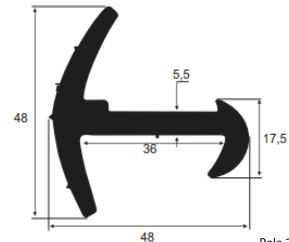
113107 SBR 80 Sh A 1113436 SBR 85 Sh A 117004 SBR 80 Sh A (barra c/ 2,80m) 117005 SBR 80 Sh A (barra c/ 2,30m) 113661 SBR 75 Sh A Vedação porta furgões
