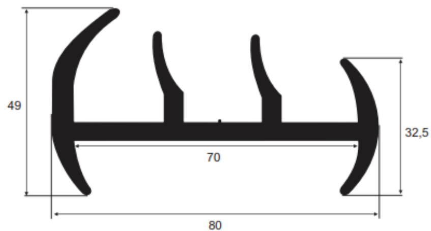
113139 EPDM 75 Sh A Vedação furgão frigorífico
