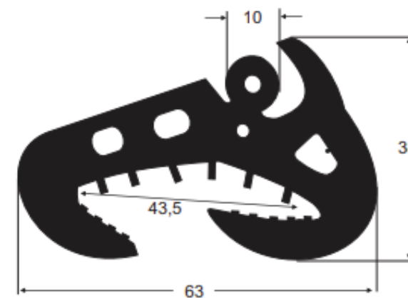
18039 EPDM 60 Sh A Janela lateral Comil- ônibus
