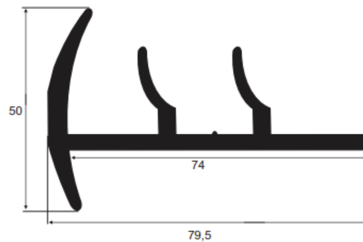
113413 EPDM 75 Sh A Vedação porta frigorífico
