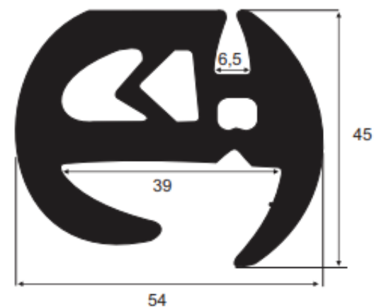
18039 EPDM 60 Sh A Janela lateral Comil- ônibus
