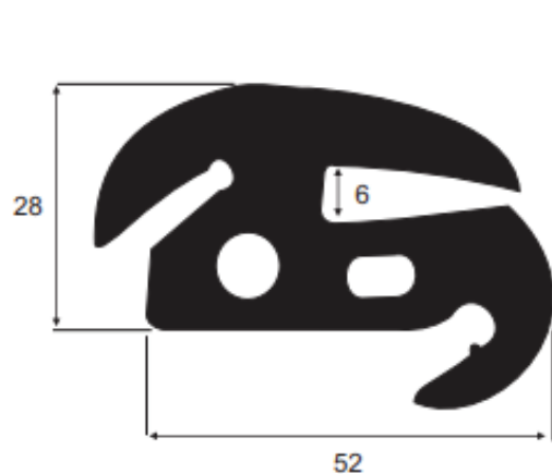
118004 SBR 60 Sh A Ved. cabine máq. agrícola
