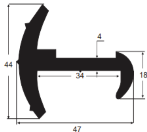
113037 SBR 80 Sh A 117008 SBR 80 Sh A (barra c/ 2,50 m) 117009 SBR 80 Sh A (barra c/ 4,60 m) 117066 SBR 80 Sh A (barra c/ 2,80 m) 117067 SBR 80 Sh A (barra c/ 2,30 m) 117075 SBR 80 Sh A (barra c/ 3,00 m) 113666 EPDM 80 Sh A Vedação porta furgões
