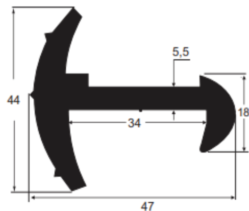
113038 SBR 80 Sh A Vedação porta furgões
